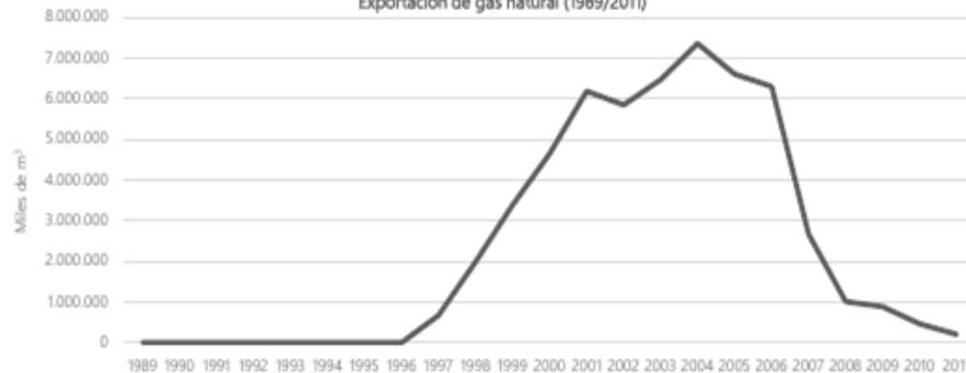
Gráfico 4.3 Exportación de gas natural (1989/2011)
