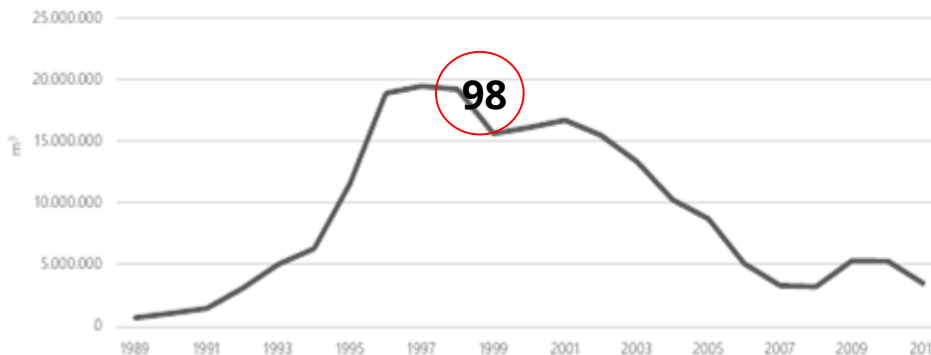
Gráfico 4.2 Exportación de petróleo crudo (1989/2011)
