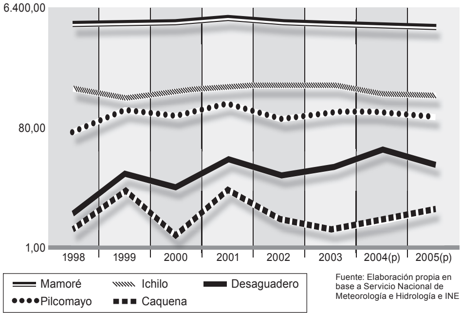
Ilustración 18. Comportamiento del caudal de ríos principales. 1998-2005
