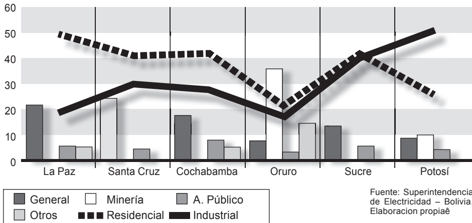
Ilustración 23. Energía facturada (MWh) de enero a septiembre 2006
