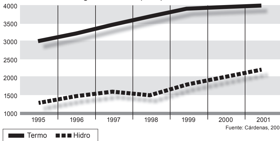
Ilustración 19. Evolución de la energía eléctrica por fuente de energía. 1995-2001 (GWh)
